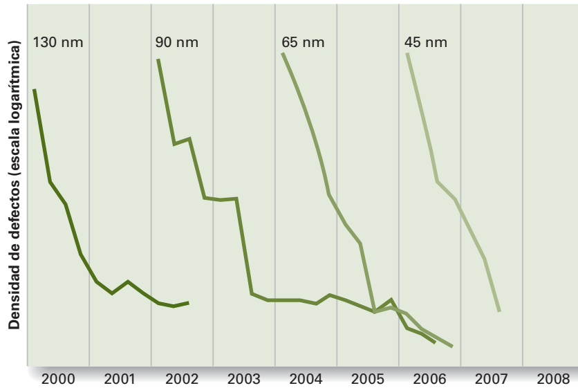
Figura 2 Rendimientos en la fabricación de microprocesadores en Intel
